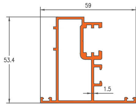
Die No. 5010 0.965Kg/m
