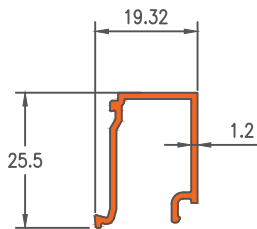
Die No. 5014 0.230Kg/m
