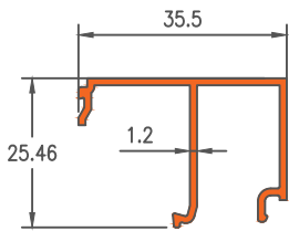
Die No. 5013 0.313Kg/m
