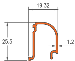
Die No. 5016 0.217Kg/m
