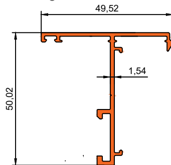
Die No. 5017 0.501Kg/m
