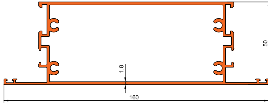
Die No. 5014 0.230Kg/m
