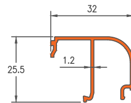
Die No. 5018 0.265Kg/m
