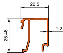
Die No. 5018 0.265Kg/m
